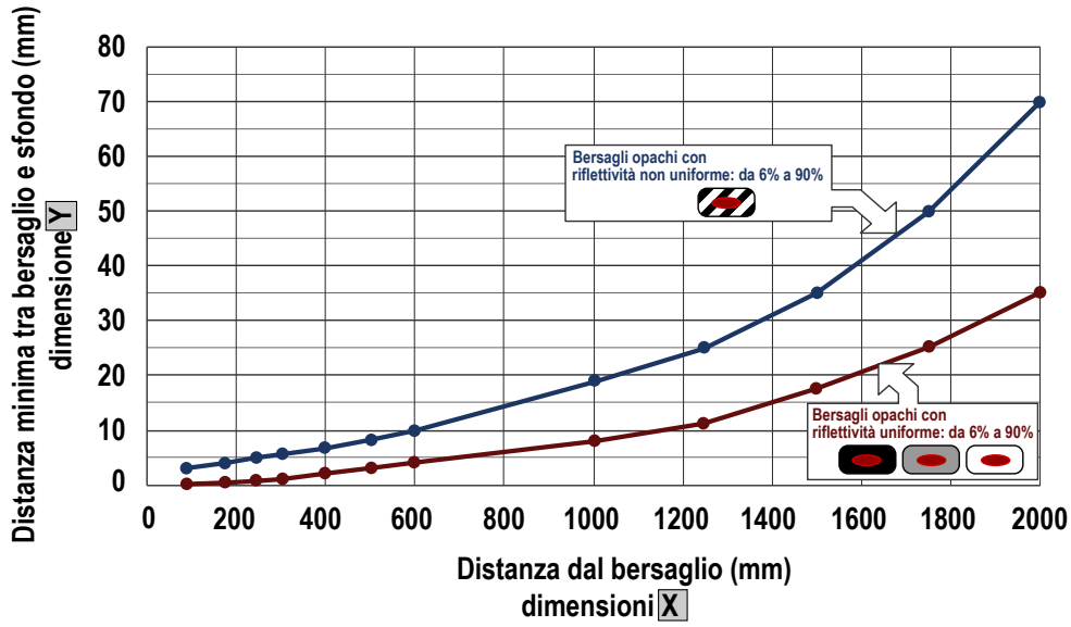
Figura 20. Prestazioni per i modelli da 2000 mm
