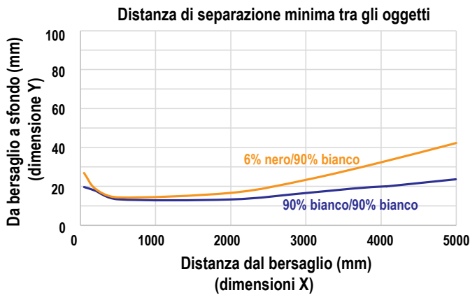
Figura 23. Distanza di separazione minima tra gli oggetti per tempo di risposta 50 ms
