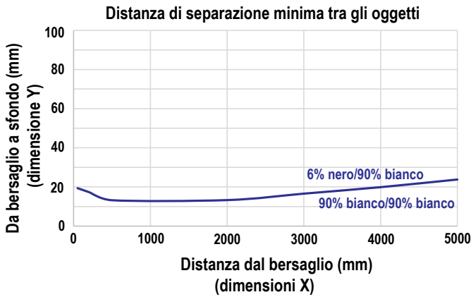
Figura 21. Distanza di separazione minima tra gli oggetti per tempo di risposta 250 ms
