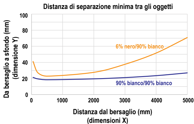
Figura 25. Distanza di separazione minima tra gli oggetti per tempo di risposta 15 ms
