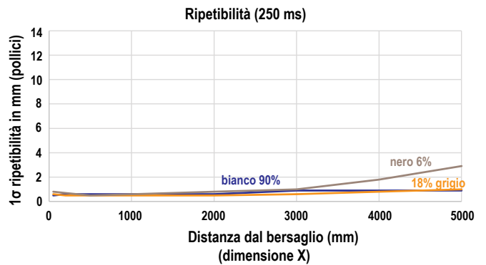
Figura 22. Ripetibilità per tempo di risposta 250 ms
