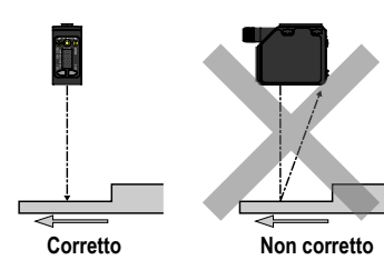
Figura 7. Orientamento per applicazioni con dislivello
