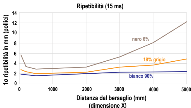
Figura 26. Ripetibilità per tempo di risposta 15 ms
