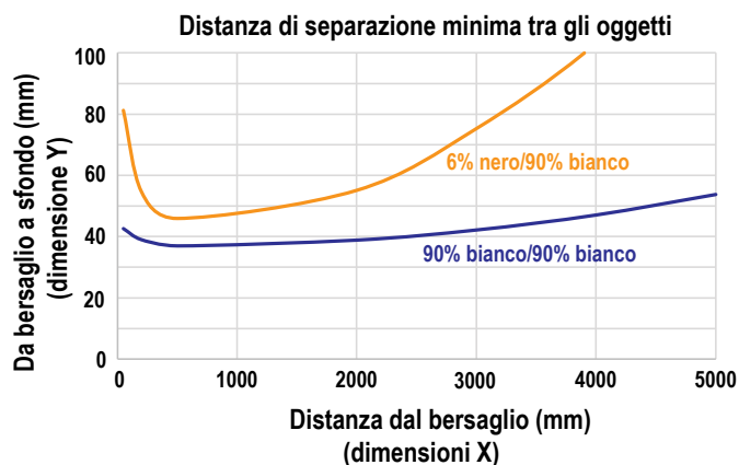
Figura 27. Distanza di separazione minima tra gli oggetti per tempo di risposta 5 ms
