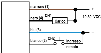
Figura 14. Canale 1 = Uscita NPN, Canale 2 = ingresso remoto NPN
