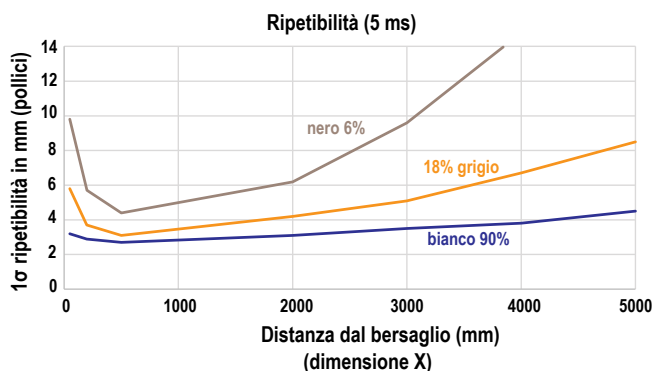
Figura 28. Ripetibilità per tempo di risposta 5 ms
