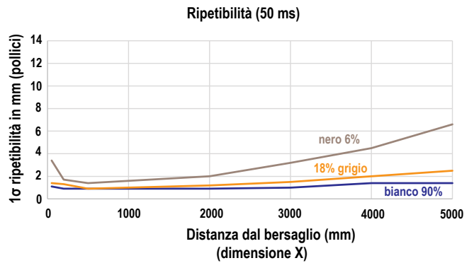
Figura 24. Ripetibilità per tempo di risposta 50 ms
