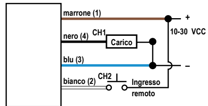
Figura 15. Canale 1 = Uscita PNP, Canale 2 = ingresso remoto PNP
